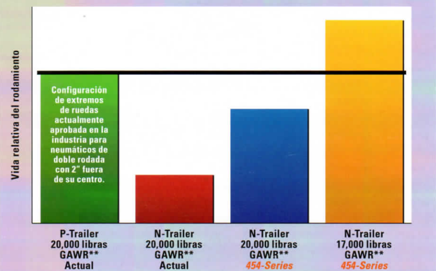
Vida de fatiga estimada del rodamiento de la rueda con neumáticos anchos de simple rodada 2" fuera del centro de carga
